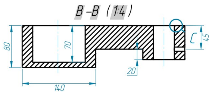
Рисунок 1.12 — Додані розміри і лінії симетрії
